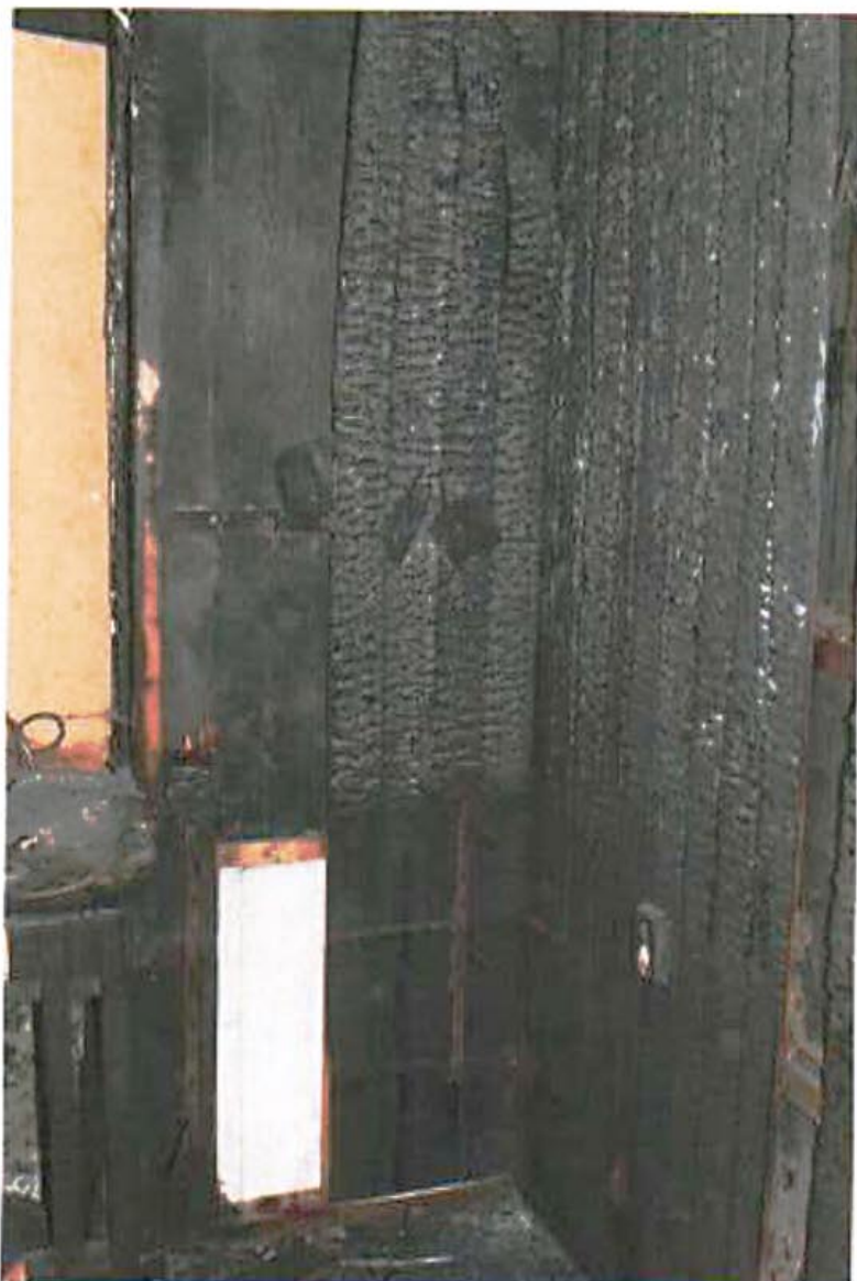
◀ Lichtbild 7 Styroporisolierung am Kopfende des Bettes
